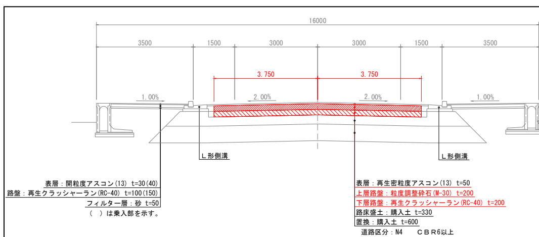
図 標準横断面図
